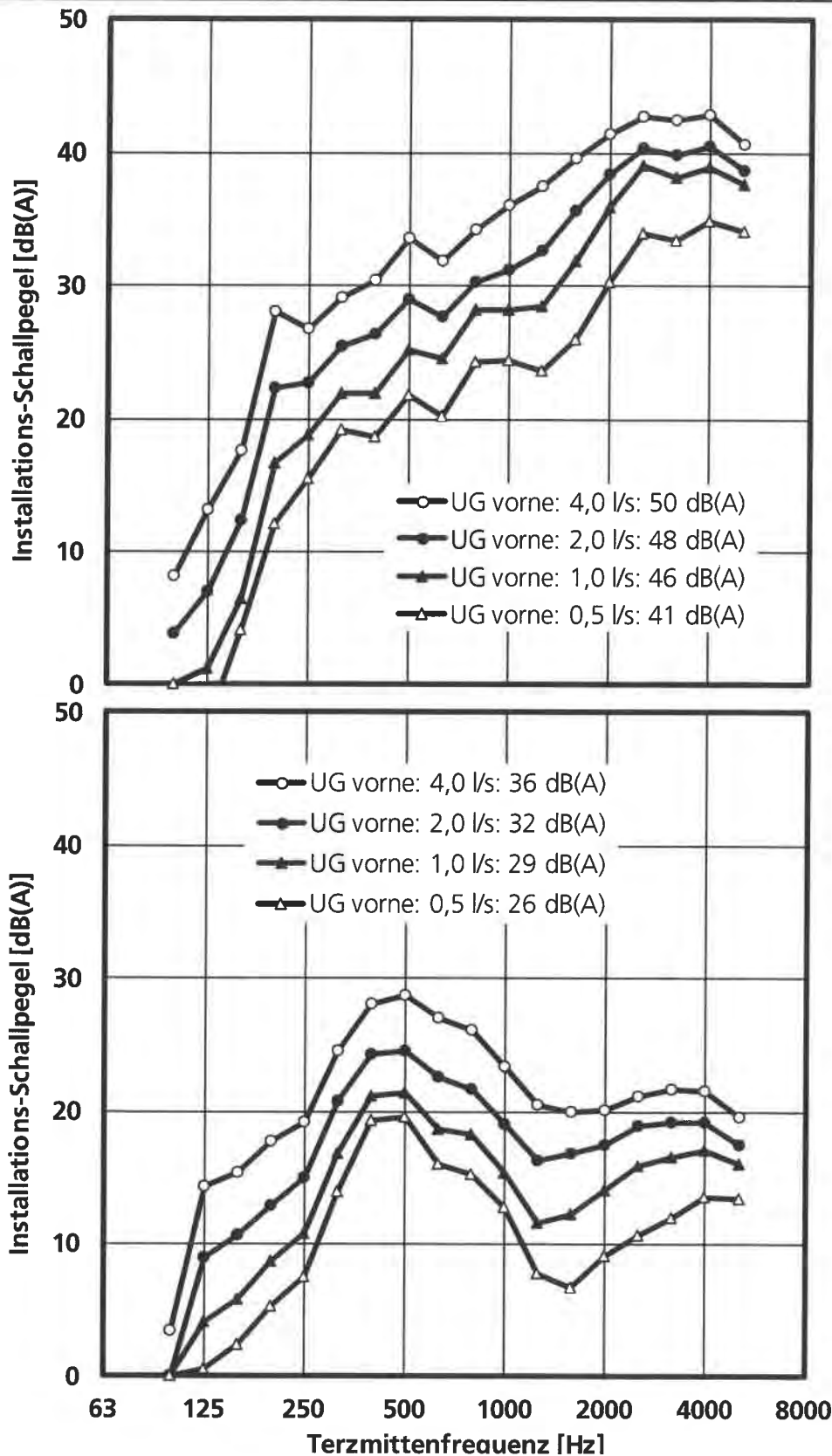
Frequenzverlauf des Installations-Schallpegels bei unterschiedlichen Volumenströmen im Installationsraum UG vorne . In der Legende sind die Installations-Schallpegel L_{A\text{Freq},n} ( L_{in} ) in dB(A) in Anlehnung an DIN 4109 für den Frequenzbereich von 100 bis 5000 Hz angegeben.
