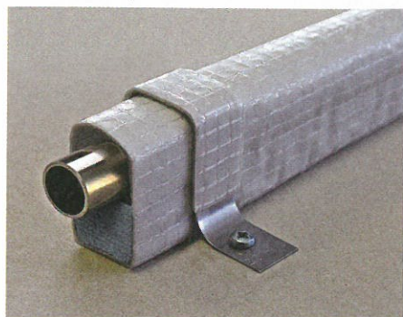
Bild 9: Mit der schallentkoppelnden Befestigung liefert Missel das intelligente Zubehör zur Dämmhülse, für die einfache und zeitsparende Montage.
