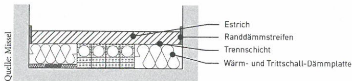
Bild 5: Das Schaubild zeigt, wie die fachgerechte Verwendung von asymmetrischen Kompakt-Dämmhülsen zu einem niedrigst möglichen Fußbodenaufbau und einem schalltechnisch sicheren Ergebnis führt.
