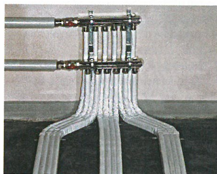
Bild 8: Kompakte Rohrtrassen auf sicherem Abstand: Praktisch umgesetzte Verlegerichtlinien mit der Missel-Kompakt-Dämmhülse an einem Leitungsverteiler
