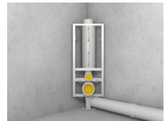
Missel-Kompakt Spülrohr MSR-M in Ecke mit Anschluss
