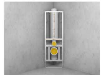
Missel-Kompakt Spülrohr MSR in Ecke mit Schallschutzprofil
