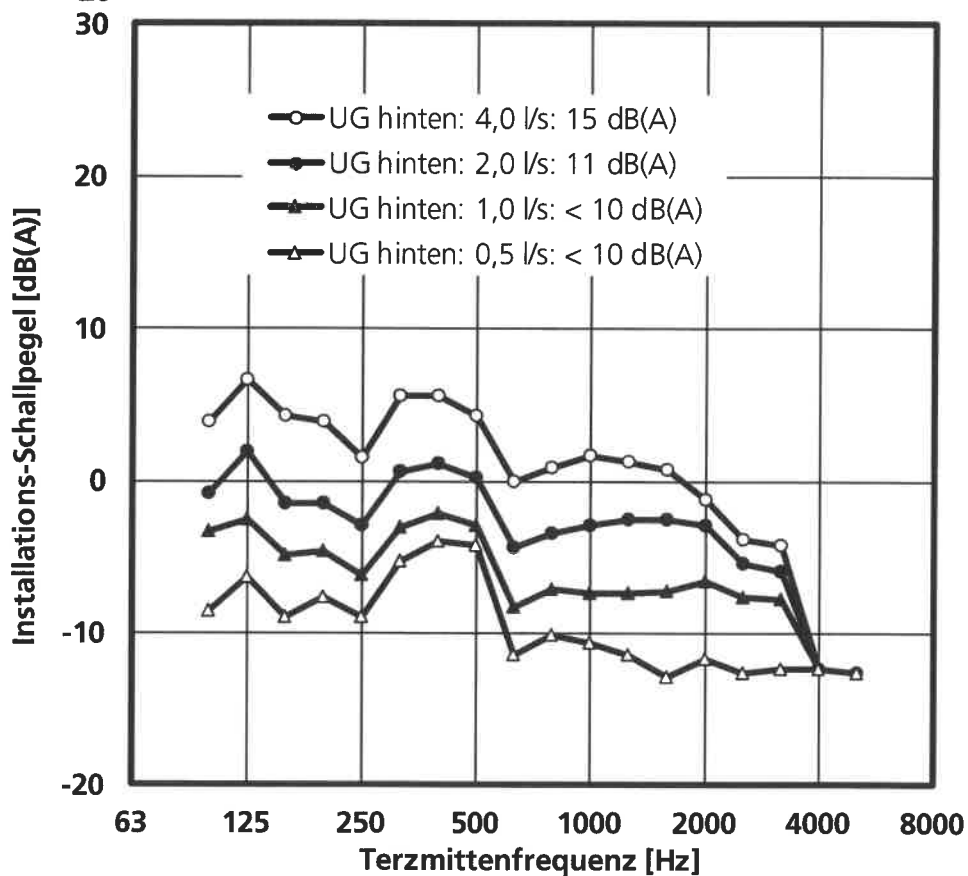
Frequenzverlauf des Installations-Schallpegels bei unterschiedlichen Volumenströmen im Installationsraum UG hinten . In der Legende sind die Installations-Schallpegel L_{A\text{Freq},n} ( L_{In} ) in dB(A) nach DIN 4109 für den Frequenzbereich von 100 bis 5000 Hz angegeben.
